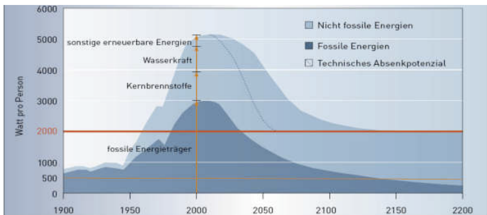
Abb. 1: Heutiger Primärenergieverbrauch pro Kopf ohne graue Energie in der Schweiz (Quelle: Kt. BE 2006)
